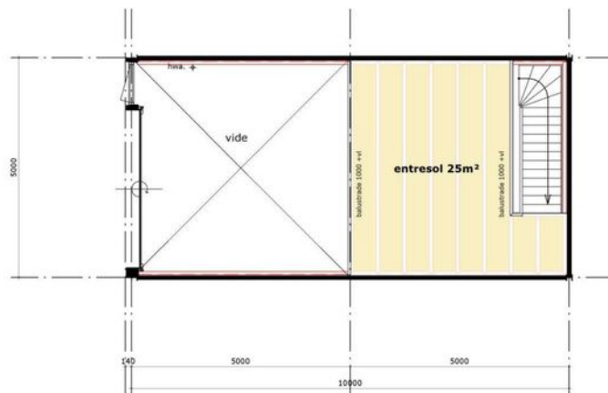
tussenvloer circa 25 m²
