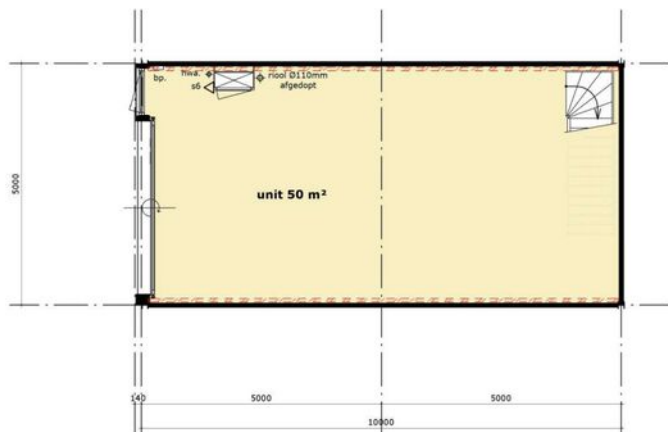
begane grond staalvoorbereiding 50 m² tussenvloer
