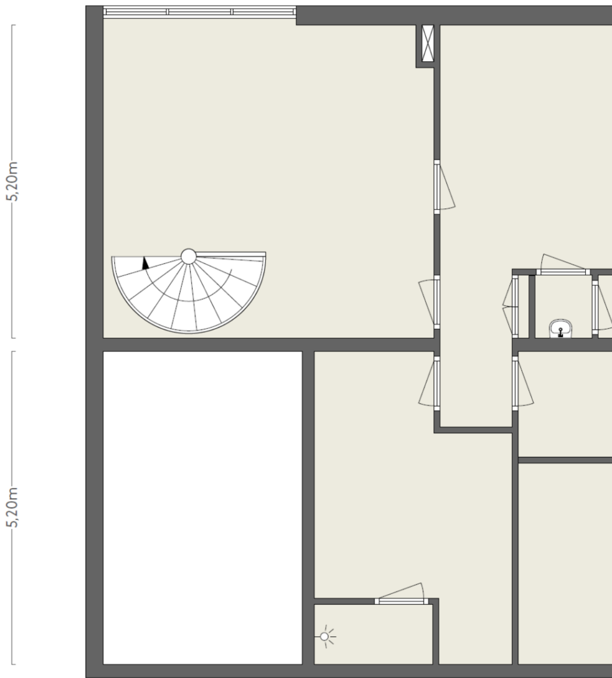
1 e VERDIEPING
