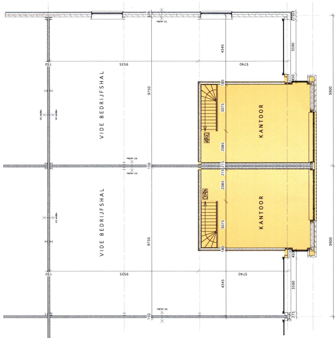
1° VERDIEPING
