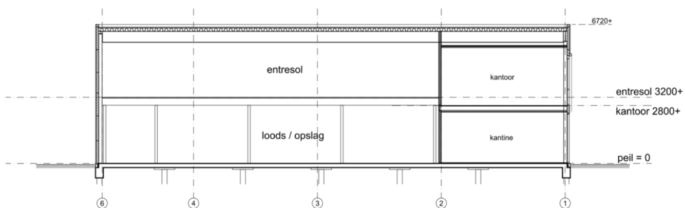
Doorsnede 2
