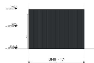
Rechterzijgezicht Unit 17
