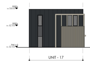
Linkerzijgezicht Unit 17
