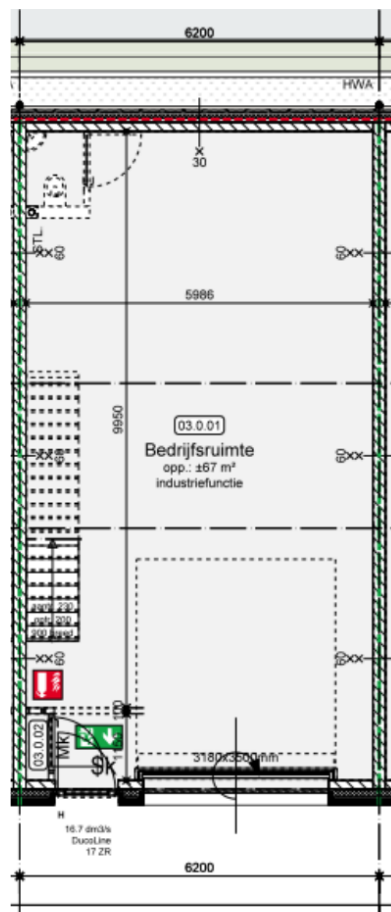
Begane grond
