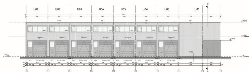
Linkergevel 2
