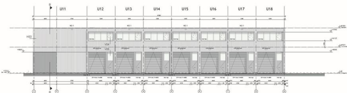
Rechtergevel 2
