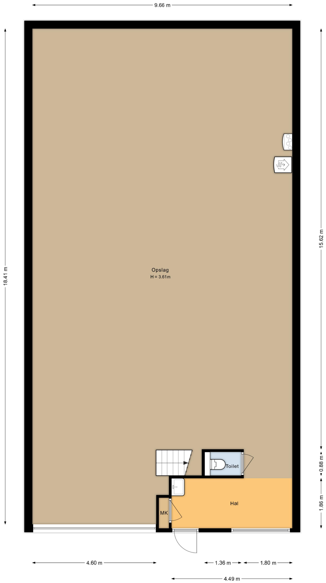
Begane grond Walserij 4 Noordwijkerhout
