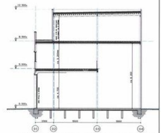
DWARSDOORSNEDE UNIT BOUWNUMMER 33
