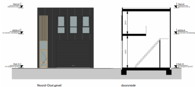
Noord-Oost gevel
