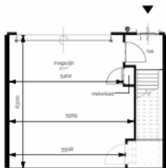
begane grond
