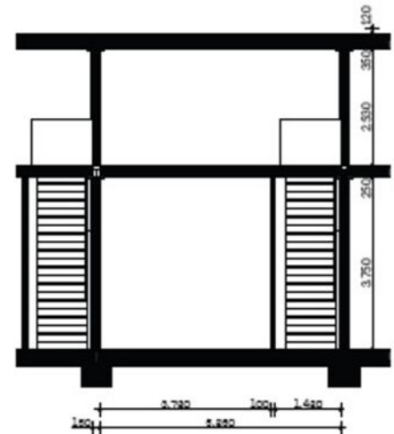
Dwarsdoorsnede - variant met gedraaide trap
