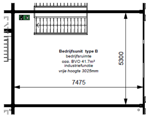
1e Verdieping
