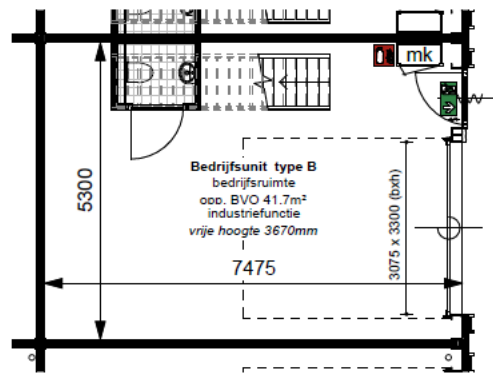
Begane grond
