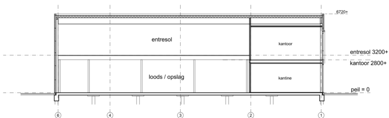
Doorsnede 2
