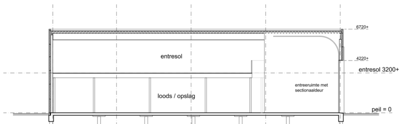
Doorsnede 2
