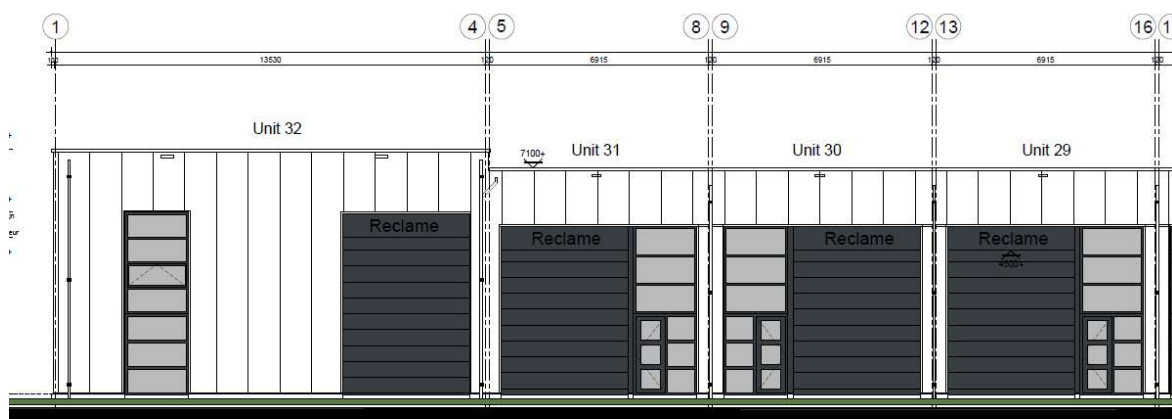
Voorgevel (zuid-west)
