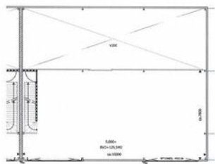
1e VERDIEPING UNIT BOUWNUMMER 33
