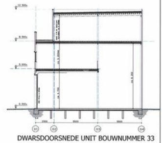
DWARSDOORSNEDE UNIT BOUWNUMMER 33
