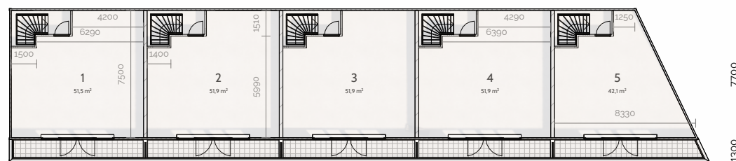
2e verdieping | BVO: 298 m²
