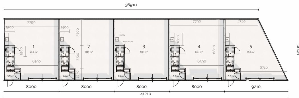
begane grond | BVO: 352 m²
