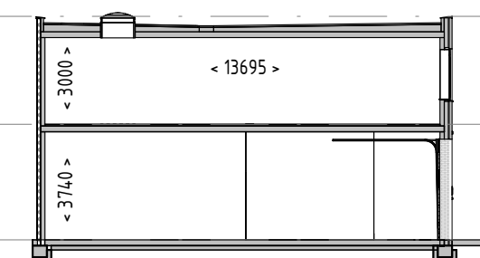
Dwarsdoorsnede
