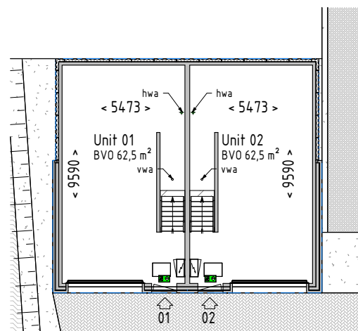
Begane grond
