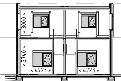
Langsdoorsnede
