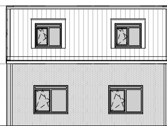
Achtergevel
