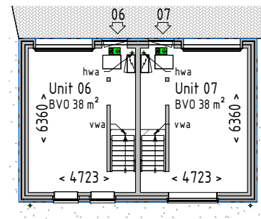
Begane grond
