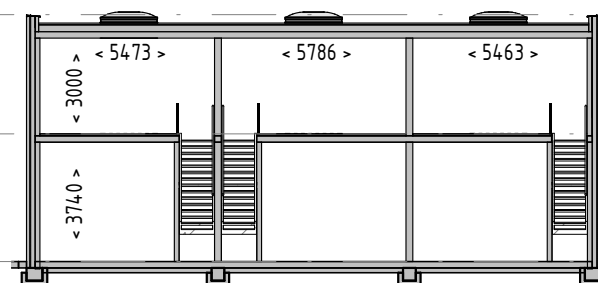
Langsdoorsnede
