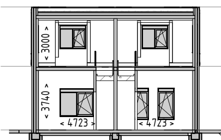
Langsdoorsnede
