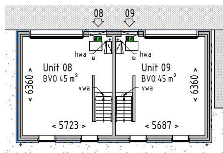
Begane grond
