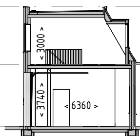
Dwarsdoorsnede
