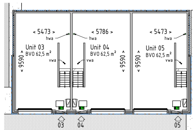
Begane grond
