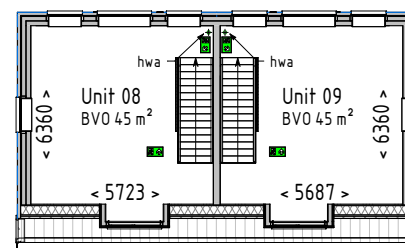
Eerste verdieping
