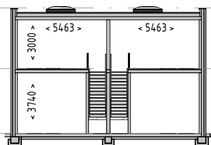
Langsdoorsnede
