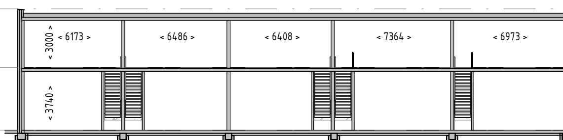
Langsdoorsnede
