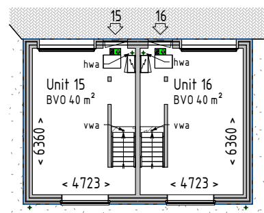
Begane grond
