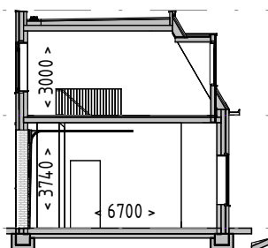
Dwarsdoorsnede
