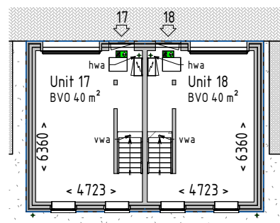
Begane grond
