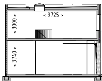
Dwarsdoorsnede
