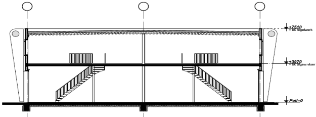
DOORSNEDE A-A
