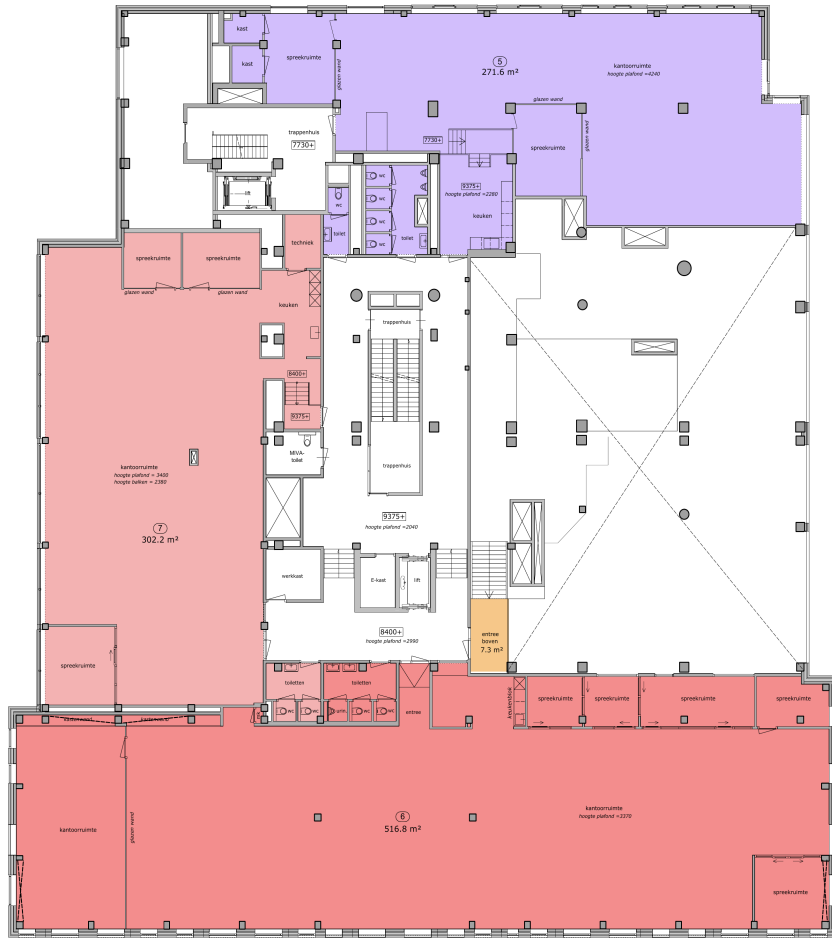
TWEEDE VERDIEPING
