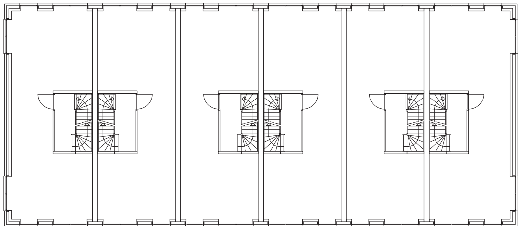
Eerste verdieping
