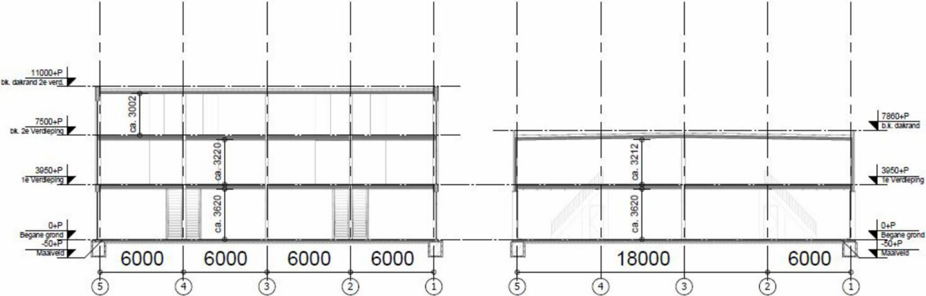
Doorsnede A
