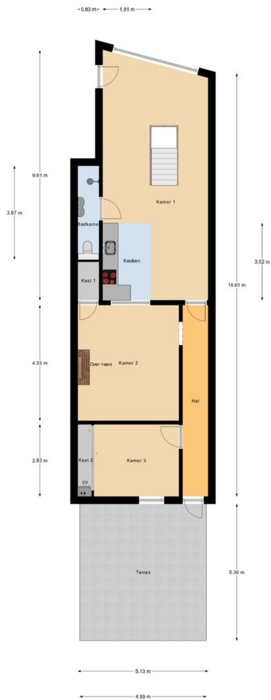
Begane Grond
