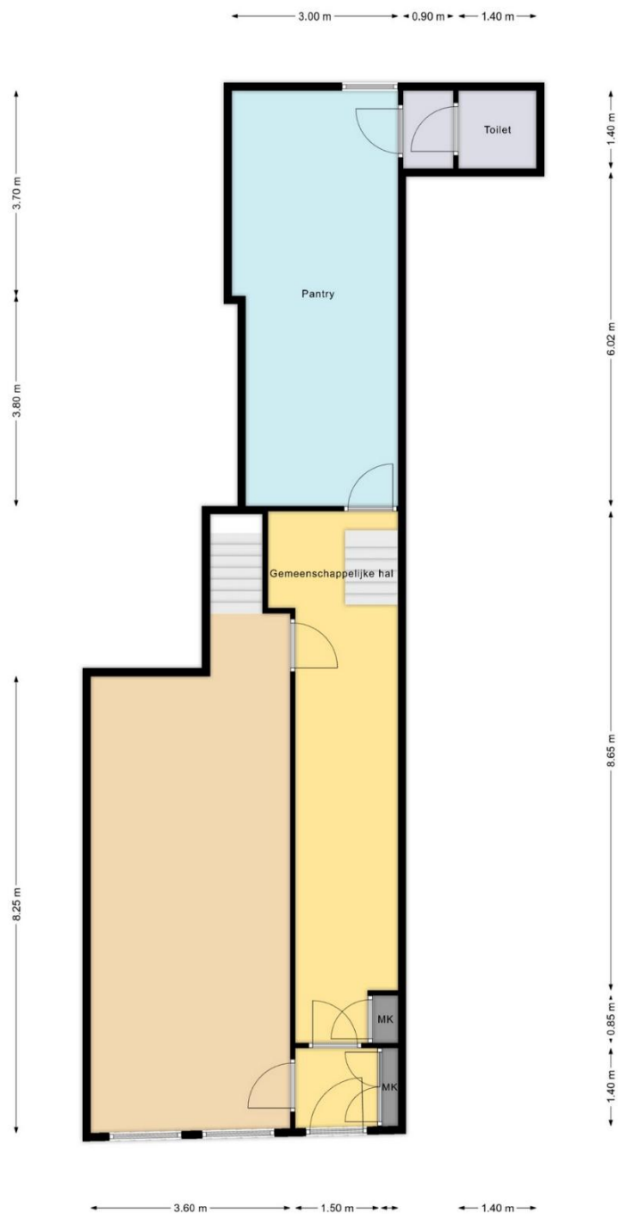
Breestraat 71 te Leiden Begane grond Indeling/maatvoering kan afwijken
