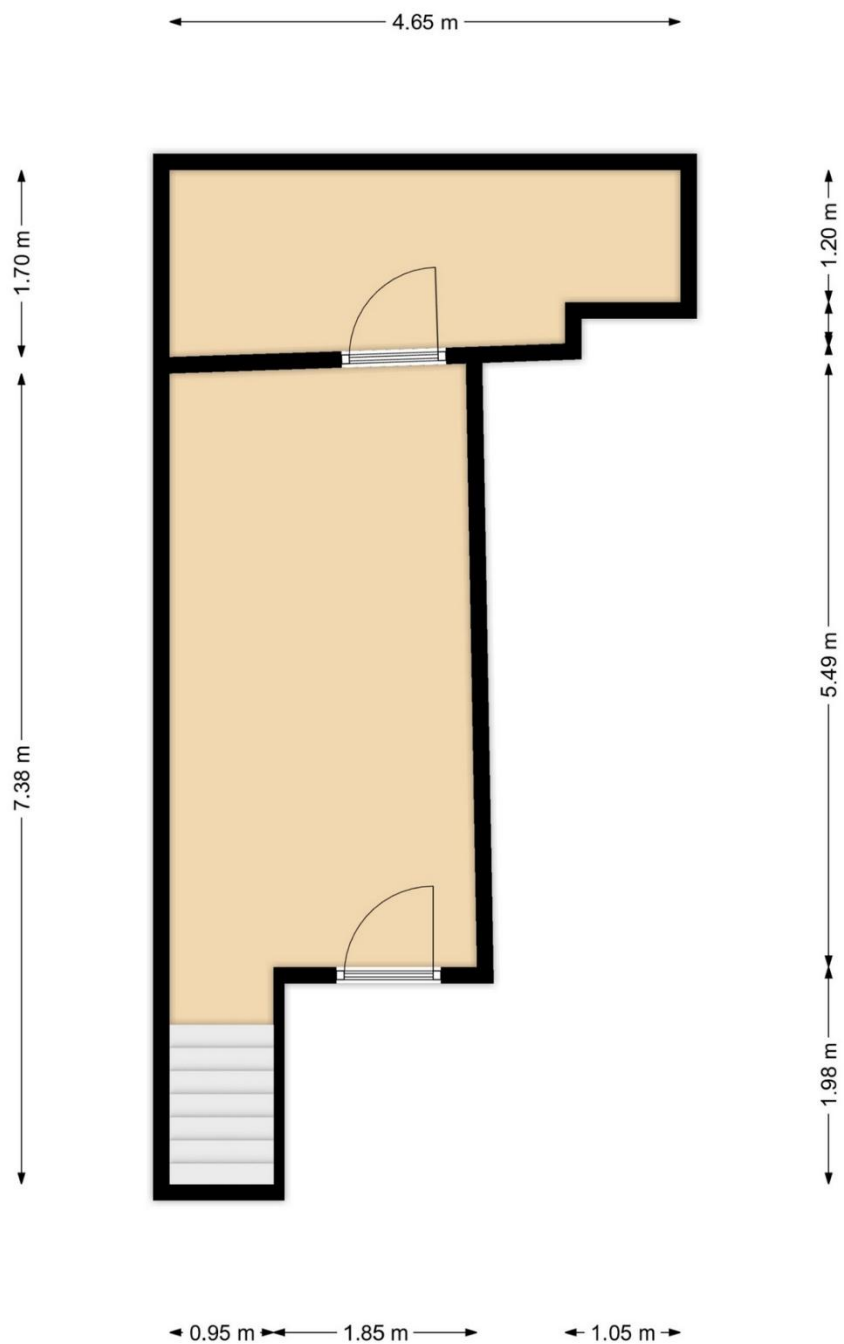
Breestraat 71 te Leiden Souterrain Indeling/maatvoering kan afwijken
