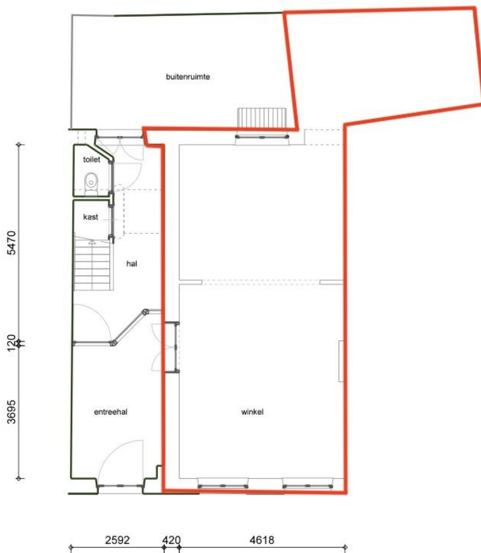
BEGANE GROND
