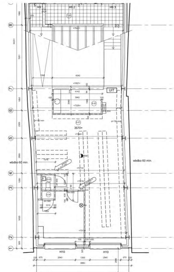
- plattegrond 2570+ / 5600+ -
