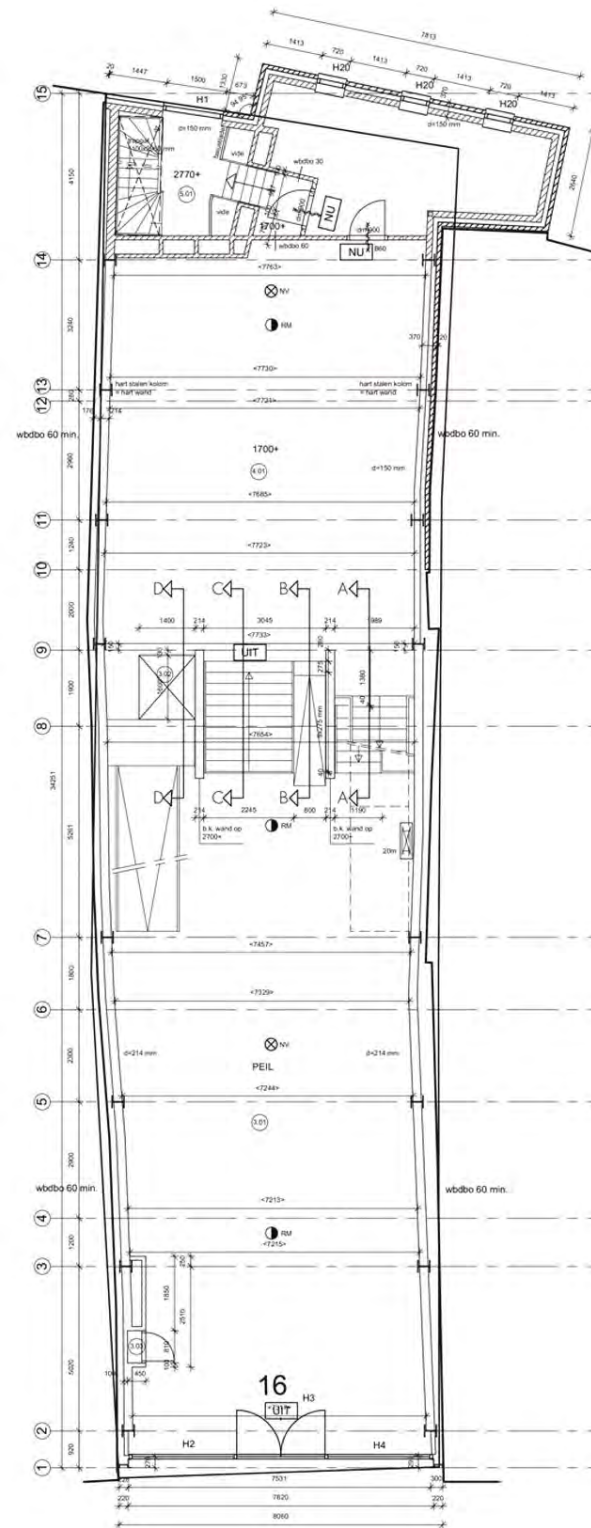
- plattegrond PEIL / 1700+ / 2830+ -
