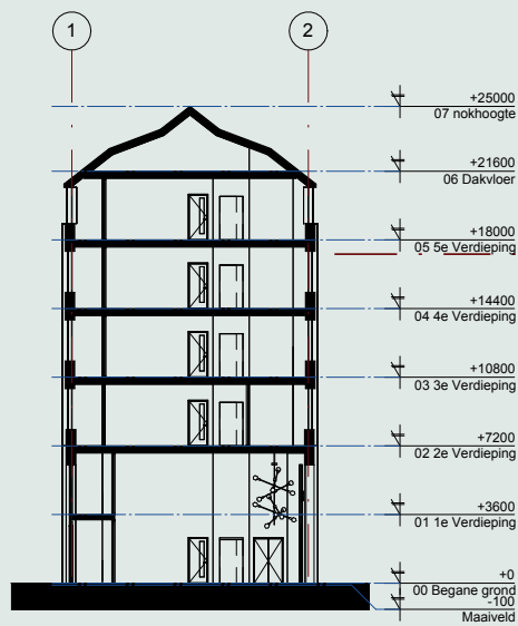
Doorsnede A-A
