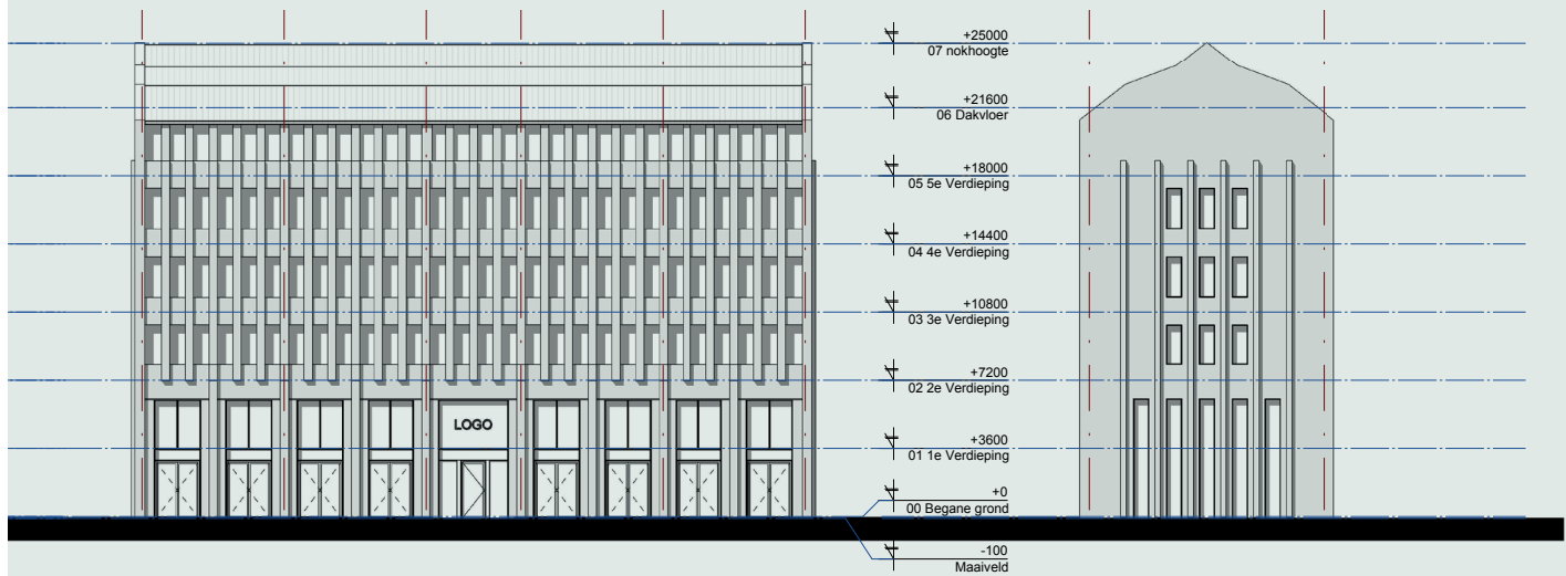
Achtergevel
