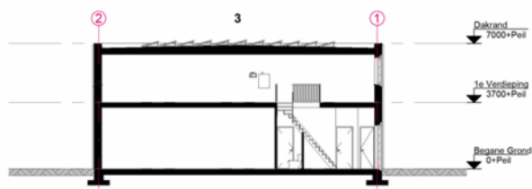
DWARSDOORSNEDE
