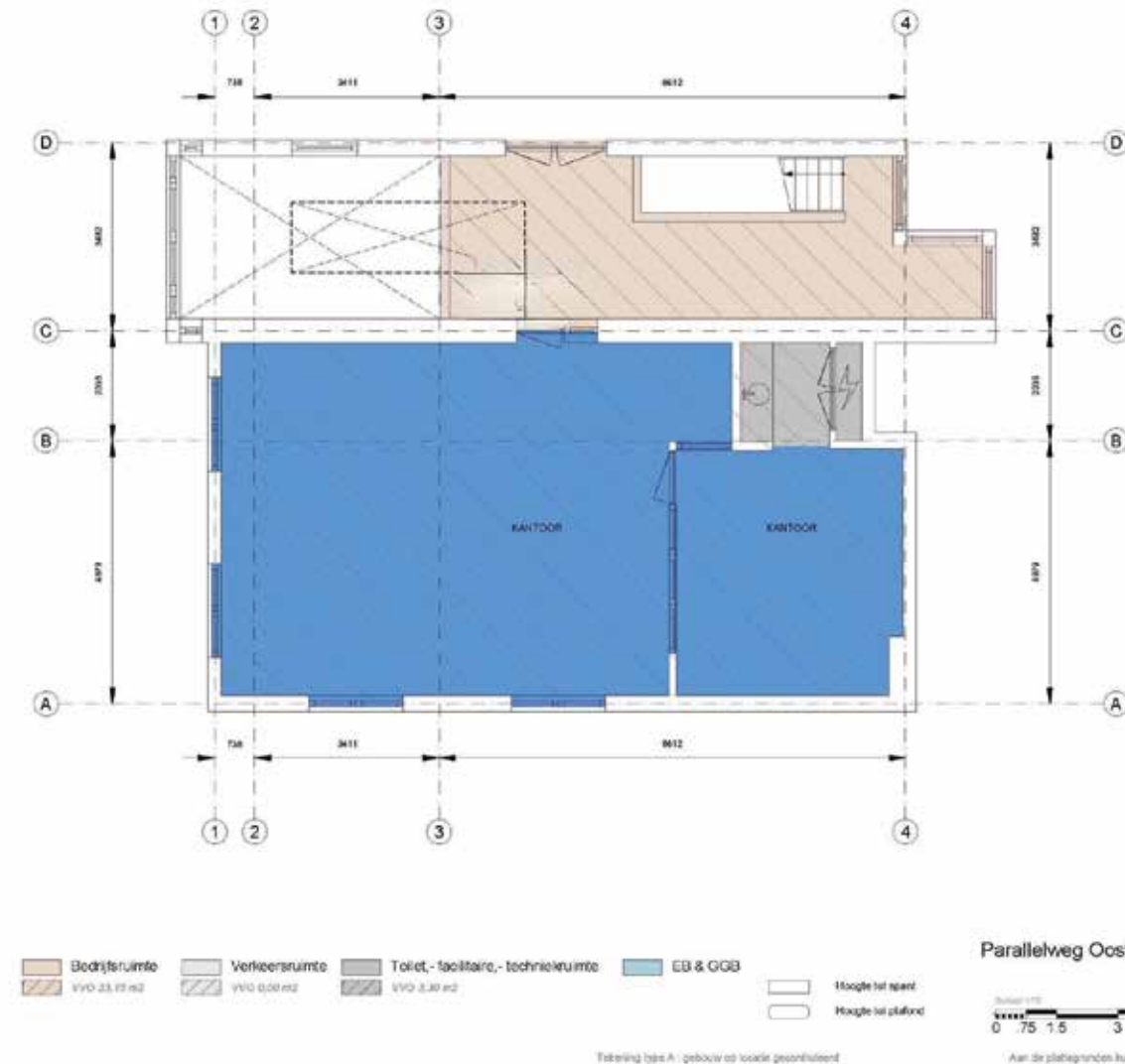
NUMMER 25 - EERSTE VERDIEPING
