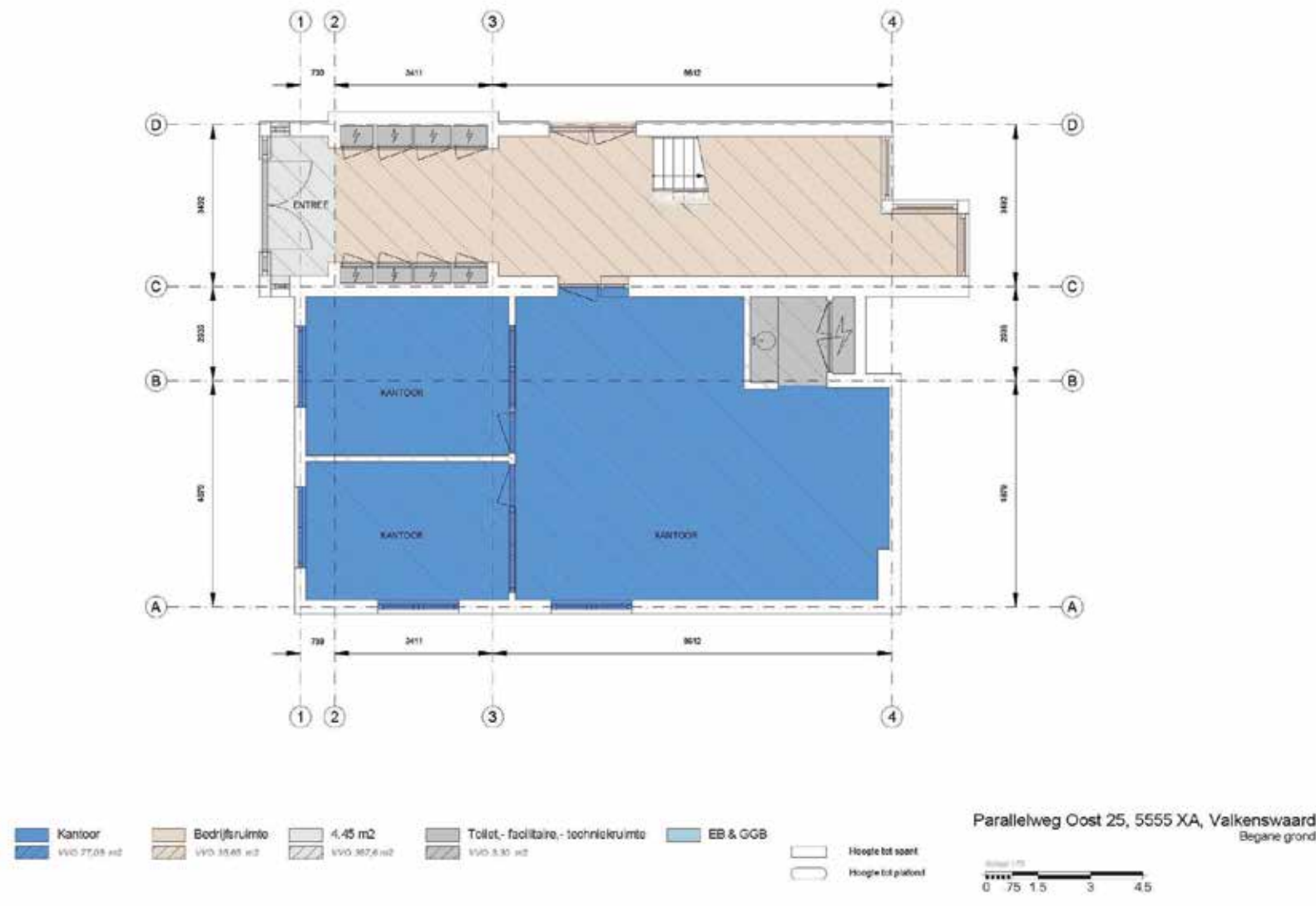
NUMMER 25 - BEGANE GROND
