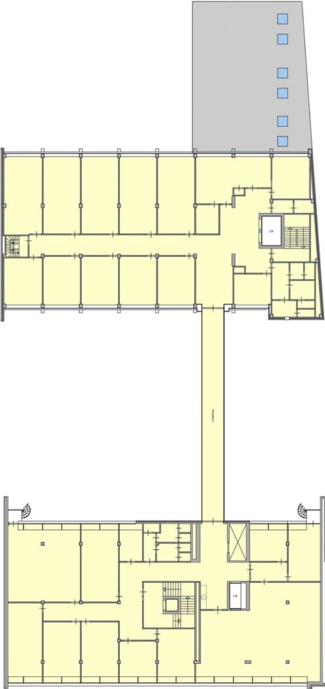
1e VERDIEPING
