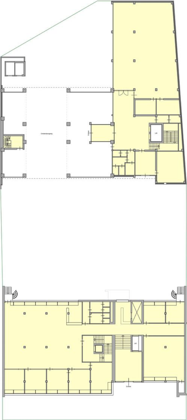
BEGANE GROND
