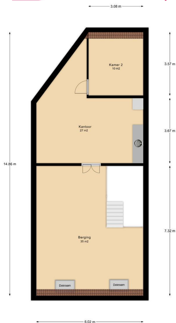
Eerste Verdieping
