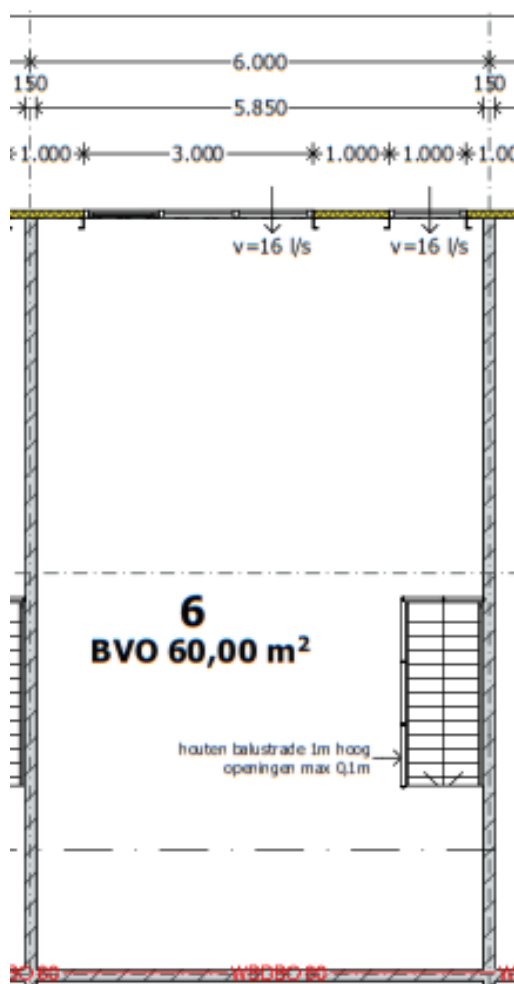
1 e verdieping
