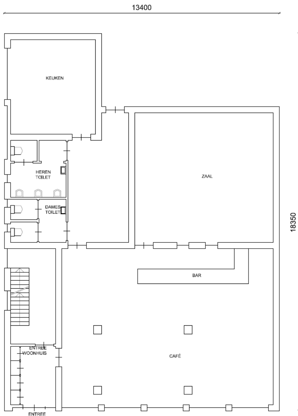
Begane Grond
