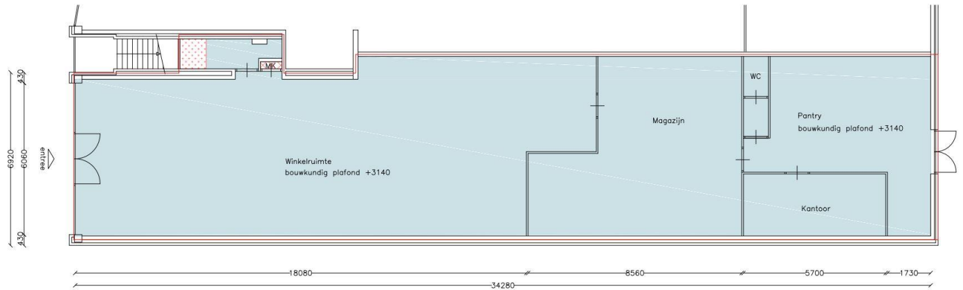
BOUWTEKENING: PLATEAU
