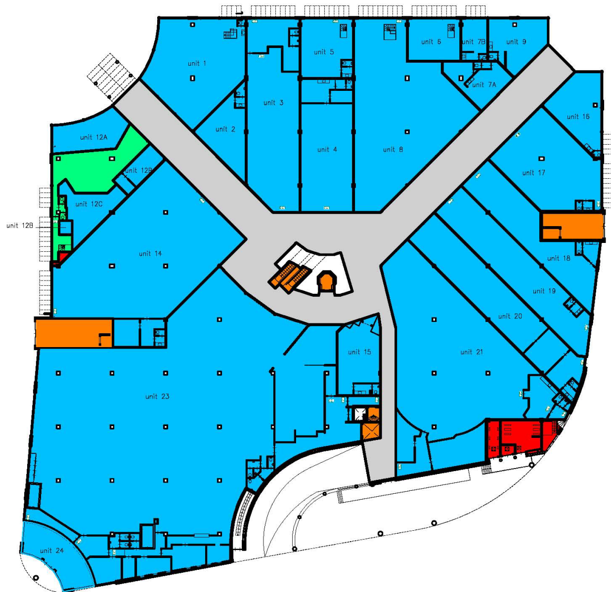
Begane grond
